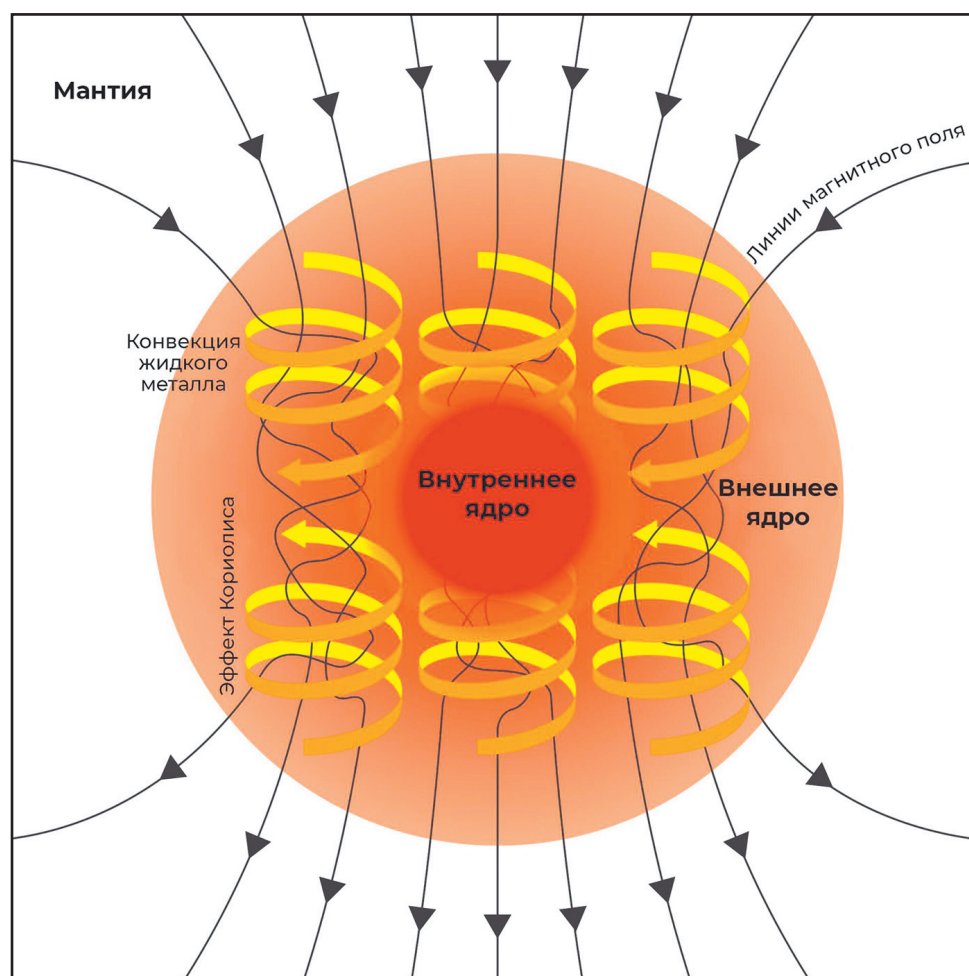
CC BY-SA 4.0 / Andrew Z. Colvin / Динамо-механизм возникновения магнитного поля Земли.
