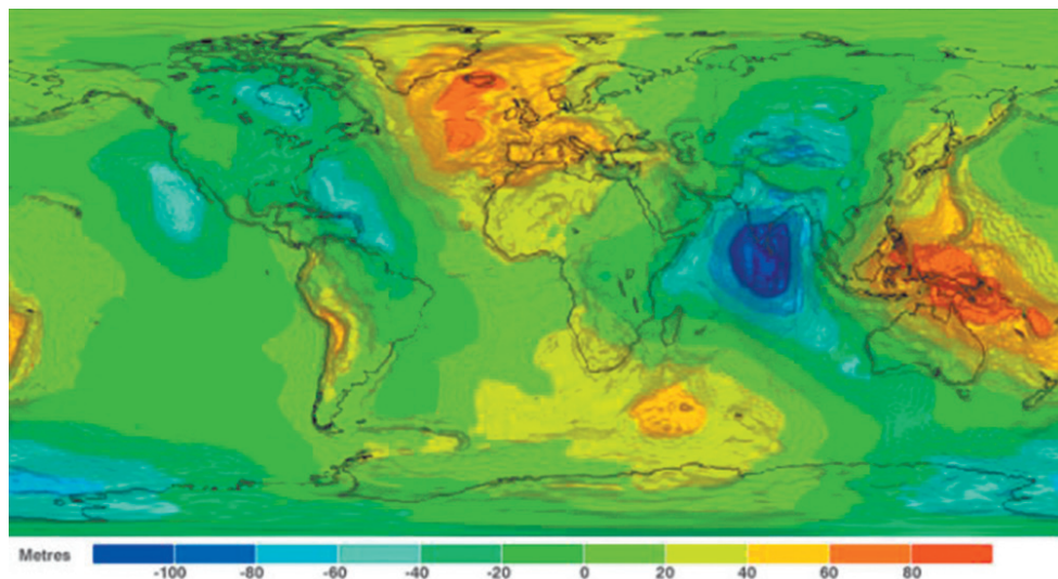
Карта гравитации Земли показывает, насколько разномасштабными являются регионы Земли по массе. Самые массивные слои в районе Исландии. Низкая гравитация у Северной Америки.
