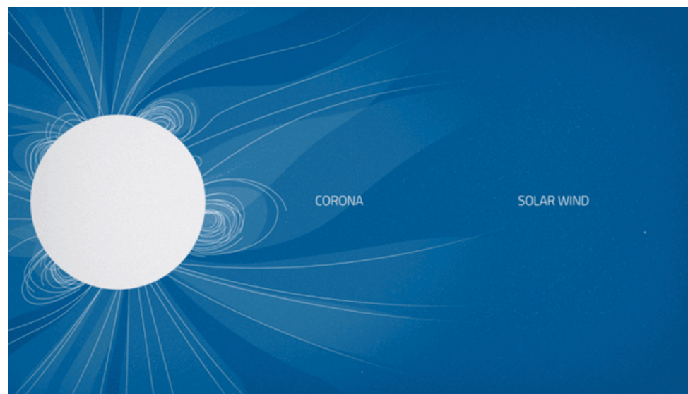
Корона и солнечный ветер (источник: https://www.nasa.gov/ )
