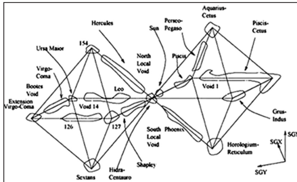
Рисунок 7.1 - Октаэдры галактик Вселенной. (E.Battaner The fractal octahedron network of the large scale structure // Astronomy and Astrophysics, v.334, p.770-771(1998)).
