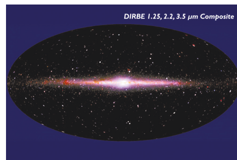
Рис. 2. Галактика Млечный Путь в инфракрасном свете, фото со спутника COBE [5].
