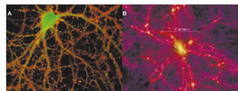
Рис. 3. Нейронные сети мозга и Вселенной: А - нейрон из гиппокампа мыши с синапсами. Зелёная клетка в центре имеет размер 10 мкм. В - космическая сеть. Длина приведённого для масштаба отрезка 1,4 \times 10^{24} м.
