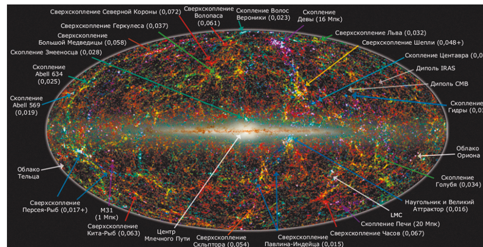
Рис. 1. Распределение галактик за пределами Млечного Пути.
