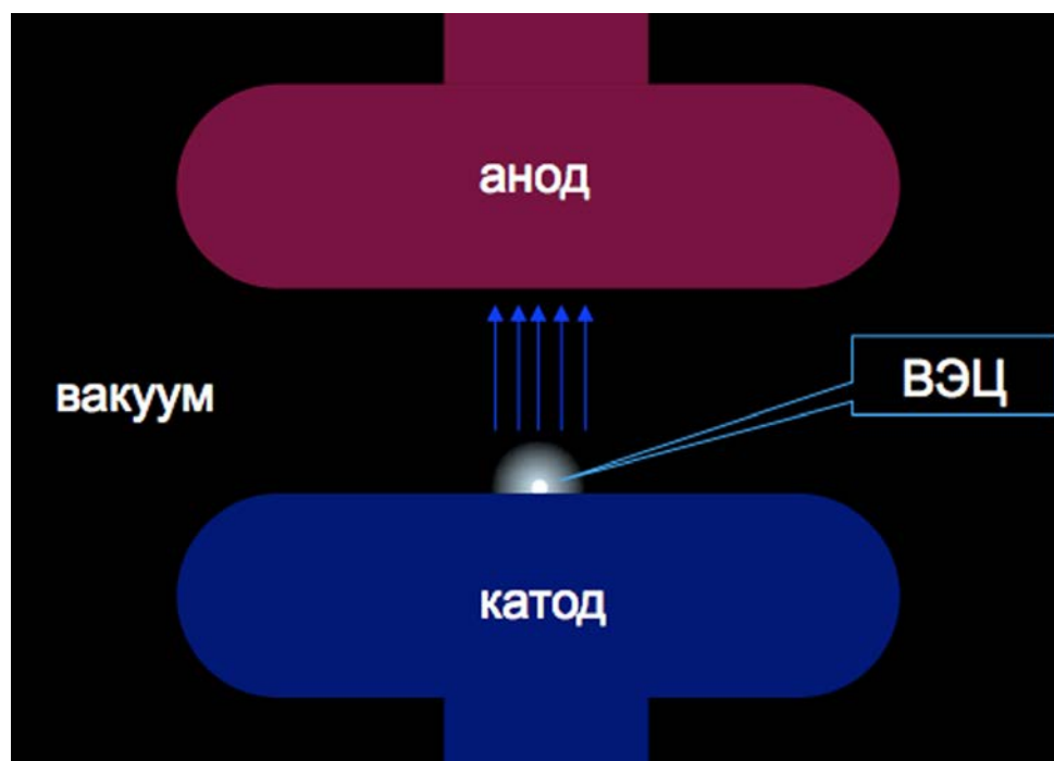
Рис. 1. Инициирование пробоя. Происходит микровзрыв эмиссионного центра (ВЭЦ). Создается «шарик» катодной плазмы, с поверхности которого эмитируются электроны в сторону анода. Это старт процесса взрывной электронной эмиссии.
