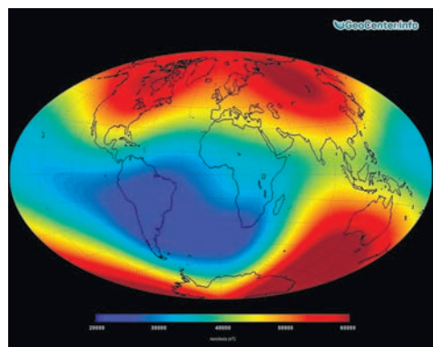
Рис. 1. «Снимок» главного магнитного поля на поверхности Земли в июне 2014 на основе данных со спутников Swarm. Красным цветом обозначены области сильного магнитного поля, а синим – ослабленного
